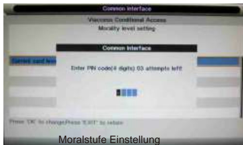
Moralstufe Einstellung
