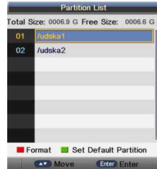
( Partitionsliste Menü)
